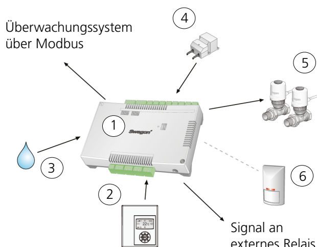
Abbildung 1. CONDUCTOR W1: Enthaltene Bauteile
