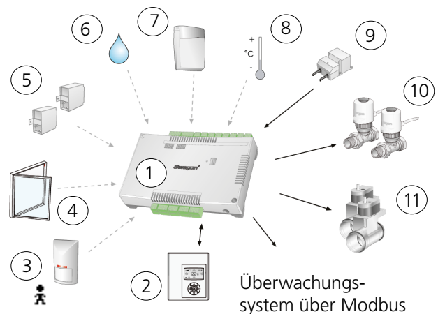
Abbildung 4. CONDUCTOR W4.1: Enthaltene Bauteile
