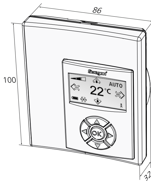
Abbildung 6. Raumeinheit CONDUCTOR RU
