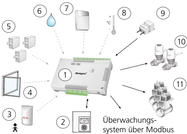
Abbildung 3. CONDUCTOR W4.2: Enthaltene Bauteile
