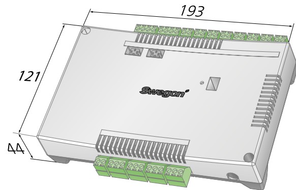
Abbildung 5. Regler CONDUCTOR RE
