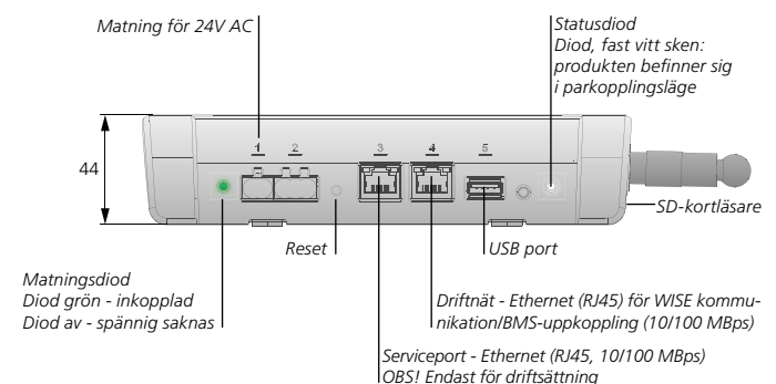
Figur 2. Kabelinkoppling och mått.
