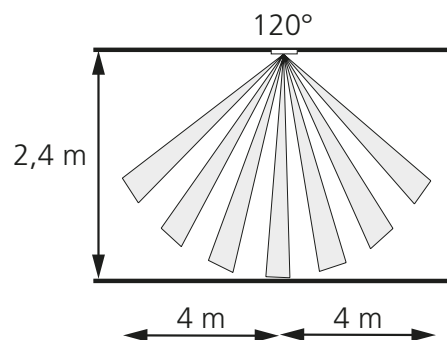
Figur 3. Detekteringsområde, takmontering.
