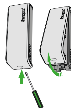
Figure 3a. Retirer la partie avant. Procéder toujours dans ce sens pour démonter le produit.
