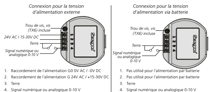
1. Raccordement de l'alimentation 0-10 V DC 2. Raccordement de l'alimentation G 24V AC / +15-30V DC 3. Terre 4. Signal numérique ou analogique 0-10 V
