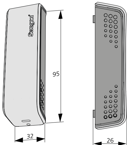
Abb. 2. Abmessungen, RTS.
