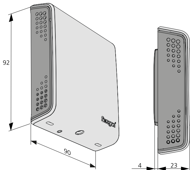
Abb. 3. Abmessungen, WISE IRT.
