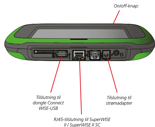
Figur 2. Tilslutninger på håndterminal TuneWISE.
