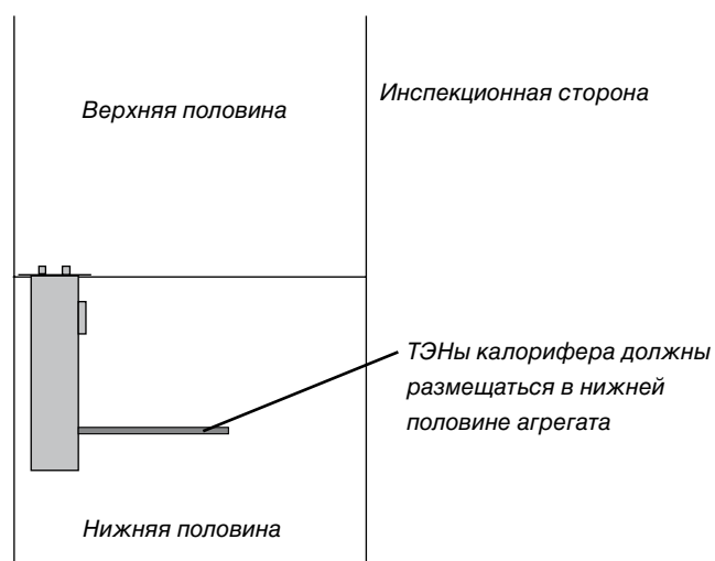
Вид агрегата сбоку
