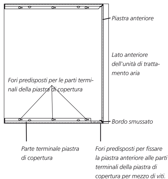
Vista dall'alto.
