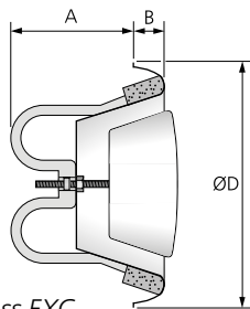
Abb. 4. Abluftauslass EXC.
