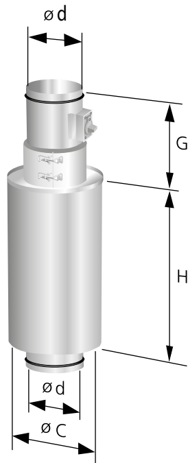
Figure 4. Unité de régulation REG.
