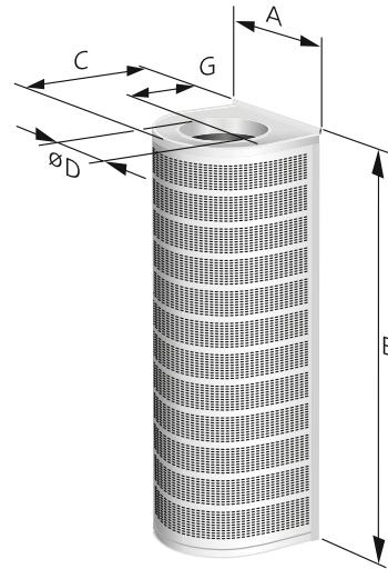
Abbildung 5. DHC
