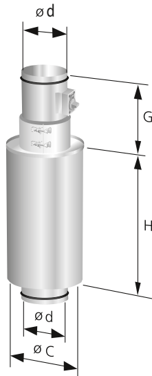
Abbildung 4. Reglereinheit REG
