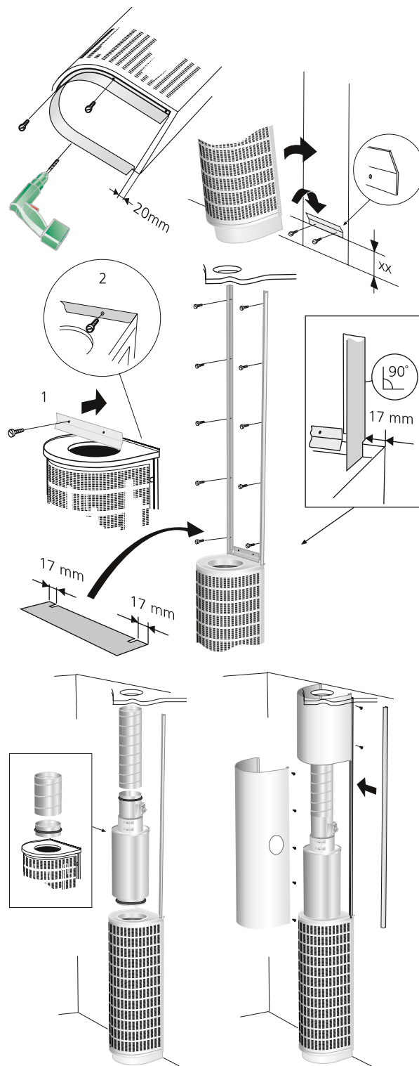
Abbildung 1. Montage
