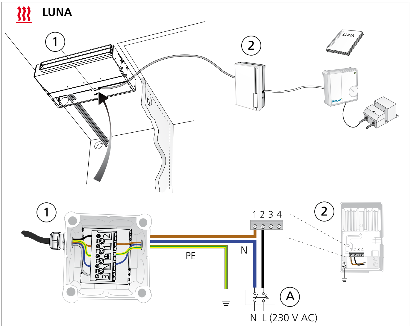
A: Allpolig brytare, brytavstånd >3mm. A: Double-pole switch, contact separation >3mm
