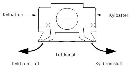
BSAb A: Kylning, ventilation
