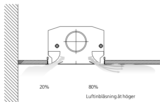
BSAb med tillval E - flödesfördelning 80/20%
