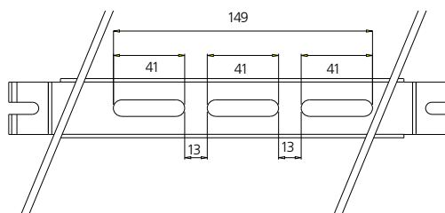
Hålbild takkonsol M10
