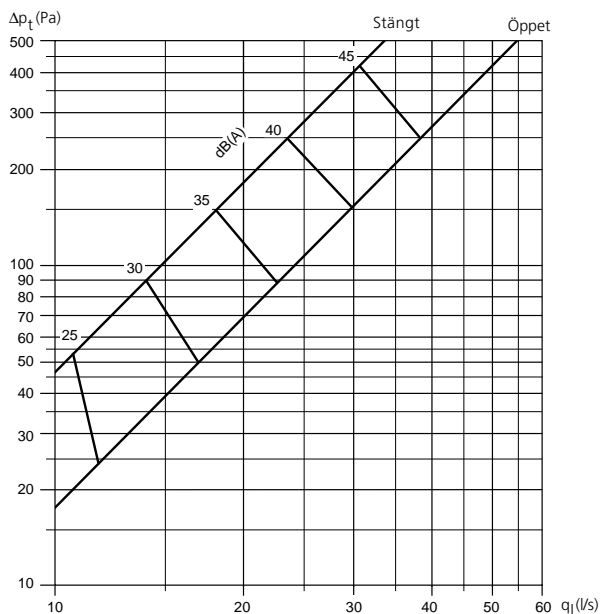
Diagram 4. Luftflöde – tryckfall – ljudnivå för L = 1,2 m
