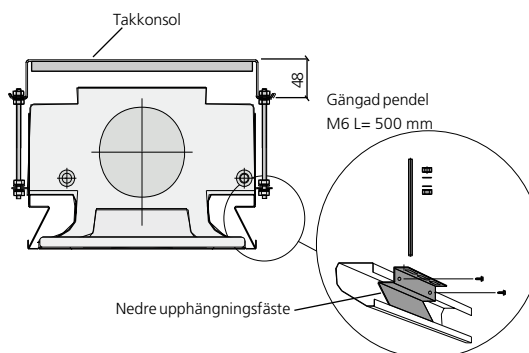
Upphängning: Montageset M10
