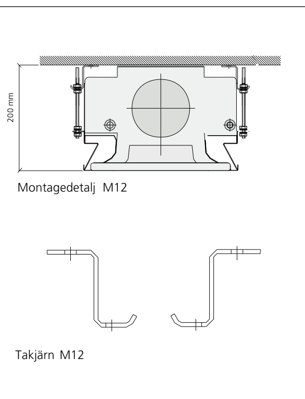
Måttabell monteringsdetalj M10S
