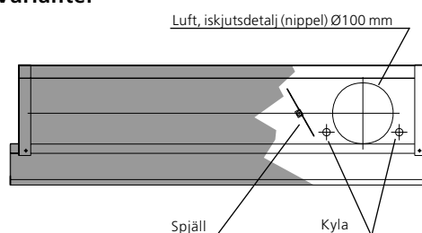
BSAb med horisontell anslutning (OH)
