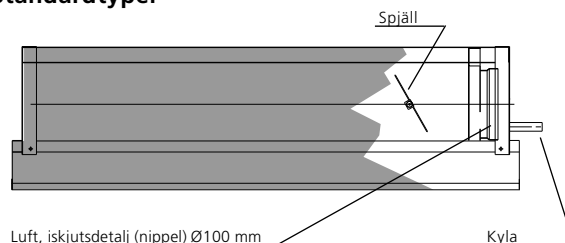
BSAb med horisontell anslutning (OH)
