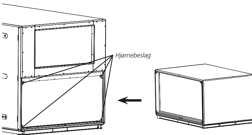
Kanaltilbehøret tilsluttes aggregatet ved at skruer medfølgende skrue+skive-sæt (4 stk.) fast gennem hjørnebeslagene fra aggregatets ventilator- eller filterrum.
