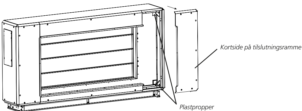
Hvis spjældet ikke er tilgængeligt til fastskruning fra nærliggende isoleret kanaltilbehør (f.eks. COOL DX, køleflade) skal den korte side på spjældets tilslutningsramme afmonteres og plastpropper fjernes, se skitsen. Så bliver spjældets monteringshjørner tilgængelige ved hjælp af et forlænget værktøj.
