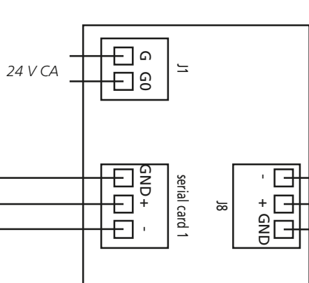
Morsetti, interfaccia di comunicazione SMART Link
