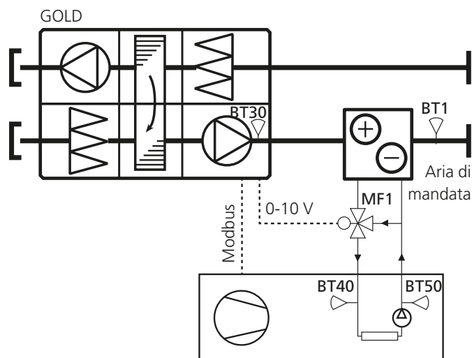
Chiller/pompa di calore Swegon È possibile aggiungere una pompa e un serbatoio di accumulo che, a seconda della taglia del sistema, possono essere all'interno o all'esterno del chiller/della pompa di calore.
