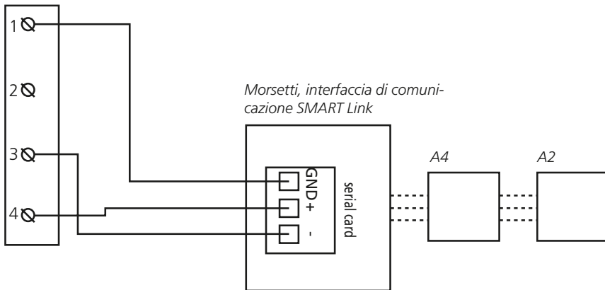
Morsetti per l'adattatore per cavi TBLZ-64
