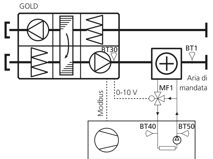
Pompa di calore Swegon
