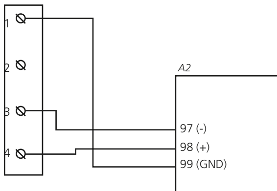
Morsetti per l'adattatore per cavi TBLZ-64
