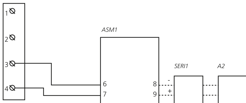
Morsetti per l'adattatore per cavi
