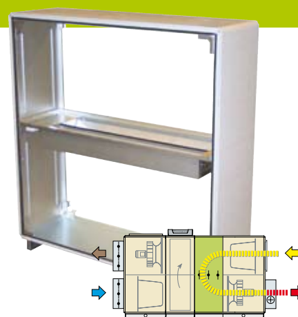
Секция рециркуляции GOLD - дешевый способ обогрева временно неиспользуемого здания, значительно снижающая расходы на его обогрев.
