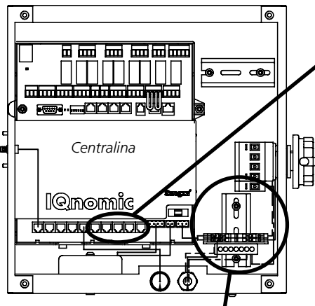
L'adattatore per cavi non è montato. Montare l'adattatore per cavi fornito all'interno dell'unità di trattamento aria GOLD senza centralina, in modo simile, in questa scatola elettrica.
