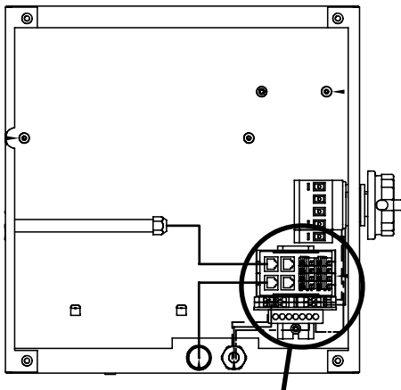
L'adattatore per cavi è montato.
