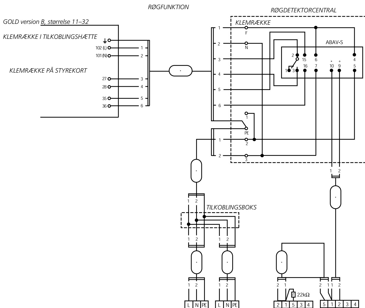
ST2:1 SPJÆLDINDSTILLINGS ANORDNING
